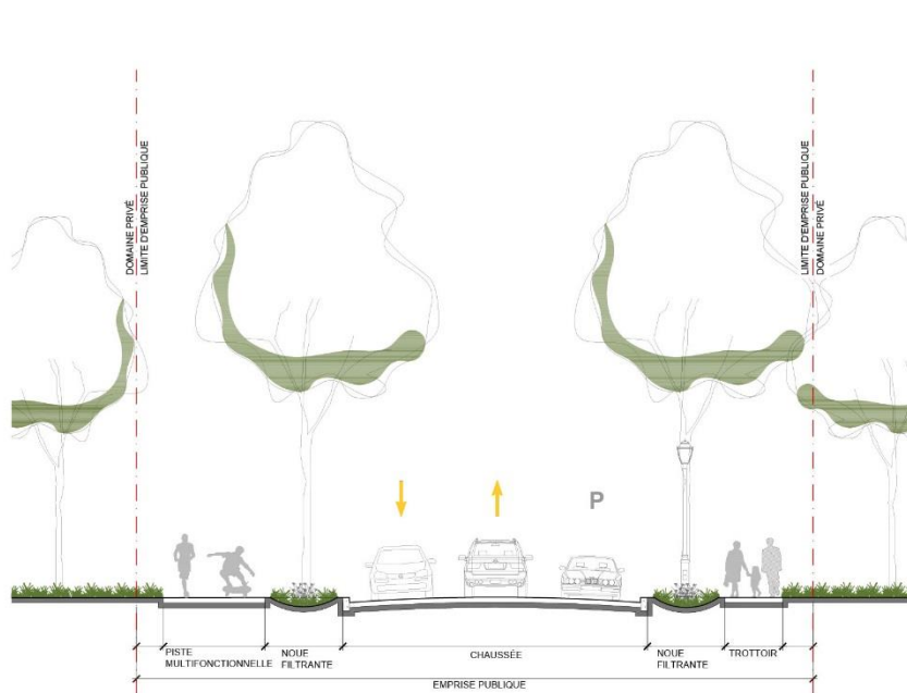
TYPE A COLLECTRICE
