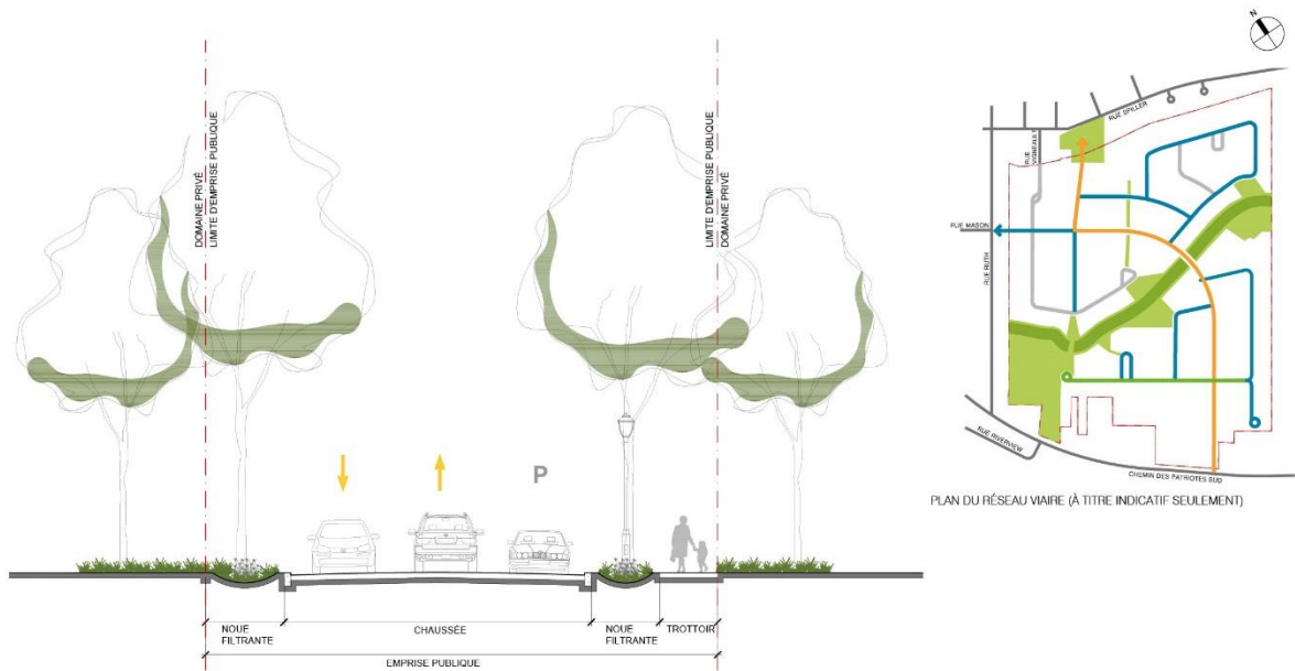
TYPE C RUE LOCALE AVEC TROTTOIR
