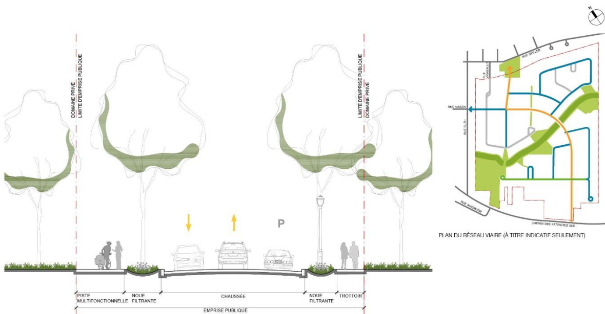
TYPE D SOUS-COLLECTRICE
