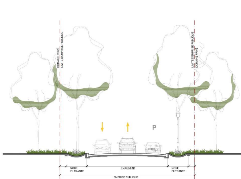
TYPE B RUE LOCALE
